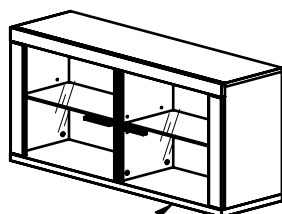
Typ 14 B/H/T 1187/549/339
